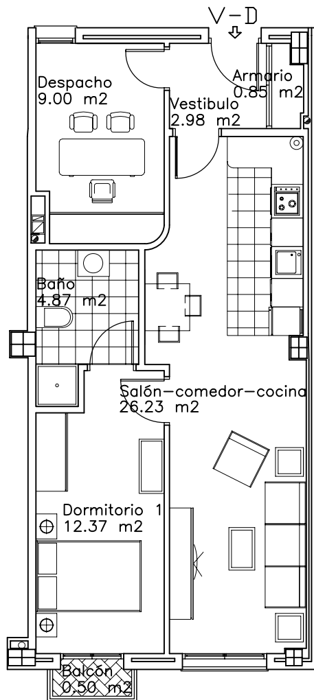
VIVIENDA D PLANTA PRIMERA, SEGUNDA Y TERCERA
